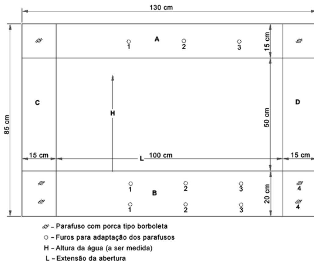
Figura 60. Vertedouro de fenda retangular.
